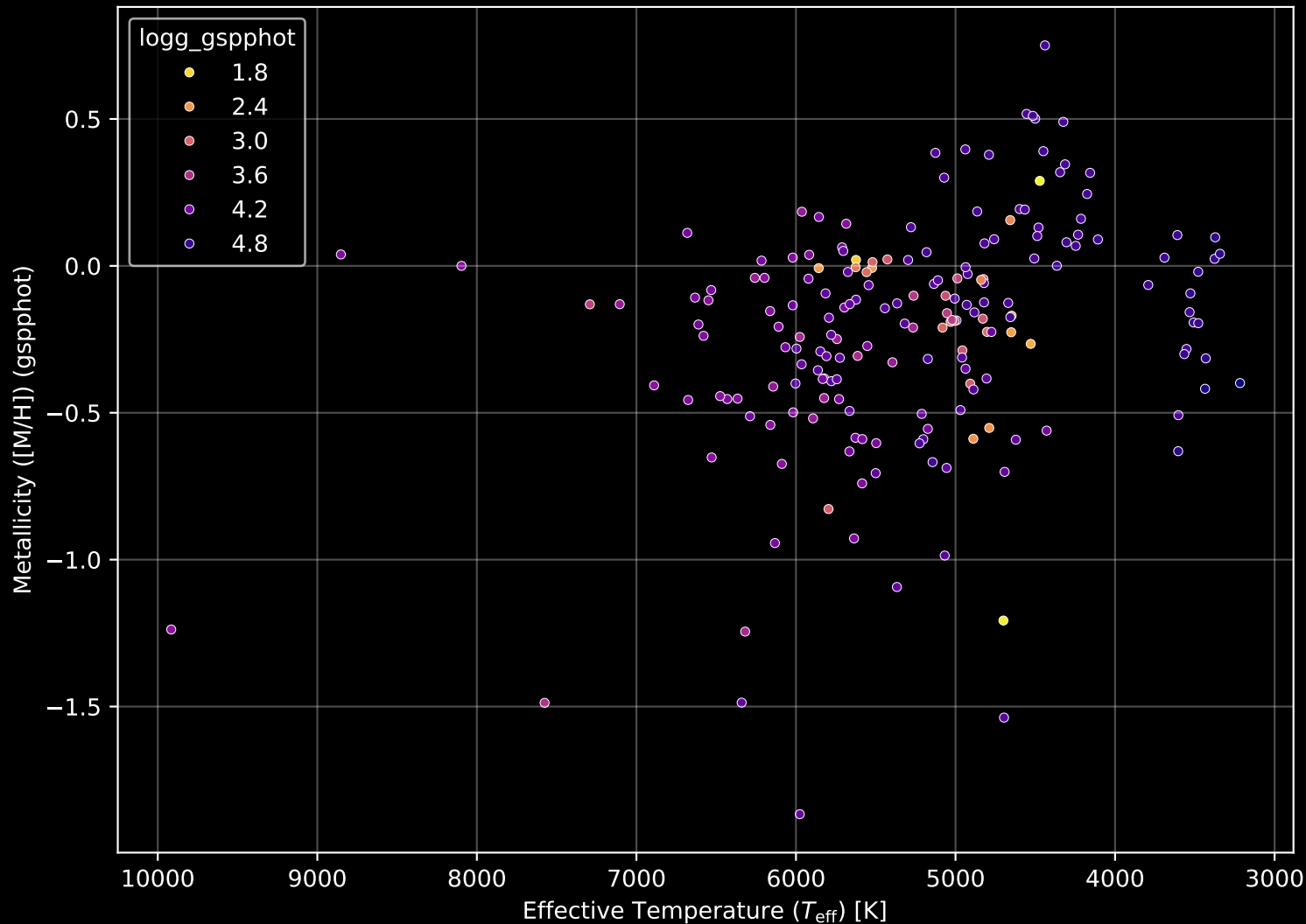
APOGEE DR17 Field: [K2_C5_215+35_btx] Stellar Population Parameters (n= 191)
